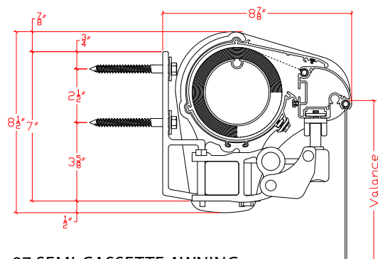
97 SEMI-CASSETTE AWNING
