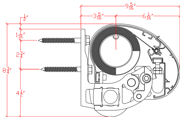
250 SEMI-CASSETTE AWNING
